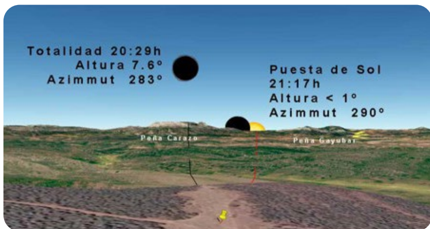
Tenada del Alto – La Luna y el Sol NO están a escala. Imagen de Google Earth y A3
